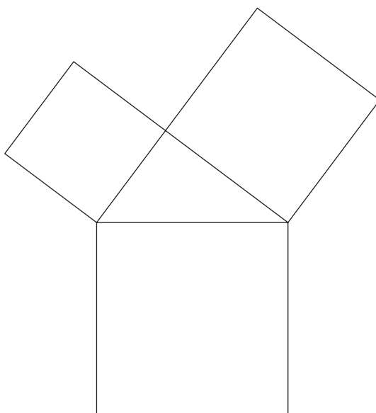
Figura 2.1: Triangolo rettangolo
