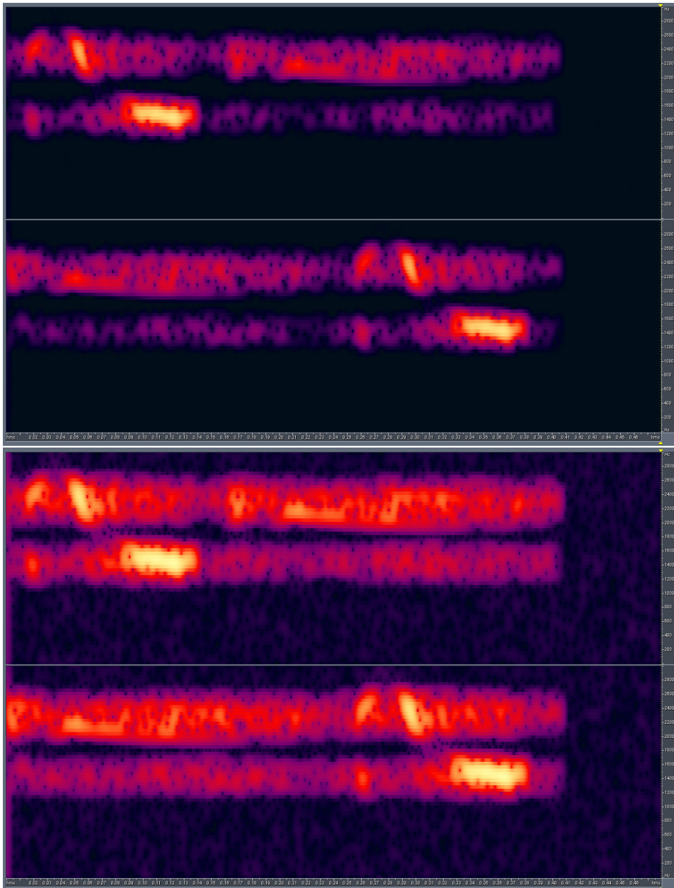
Figura 6.1: El espectro de frecuencias de los sonidos usados en este experimento (ver sección 5.4), filtrados tal como lo hacen los sensores (frecuencias alrededor de los 2293 Hz y 1392 Hz), con dos diferentes intensidades de color en la representación de la intensidad con el objetivo de observar por una parte el ruido y por otra la intensidad de la señal que usa el individuo.
