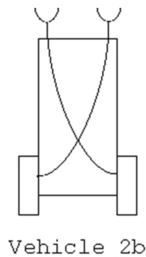
Figura 2.1: Vehículo de Braitenberg 2b.
