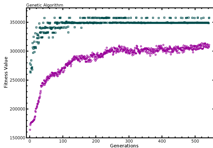
Figura 5.7: Maximos y medias de los valores de la funci3n de adecuaci3n (eje Y) de los individuos de cada generaci3n (eje X) en una ejecuci3n del algoritmo gen3tico para el experimento que tiene ruidos de fondo. Comparar con la figura 5.2.
