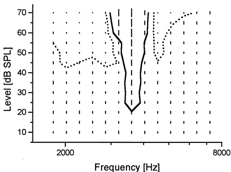
Figura B.3: Activación de una neurona sensora de estornino para cada frecuencia y volumen del sonido. Figura de Nieder y Klump (1999)
